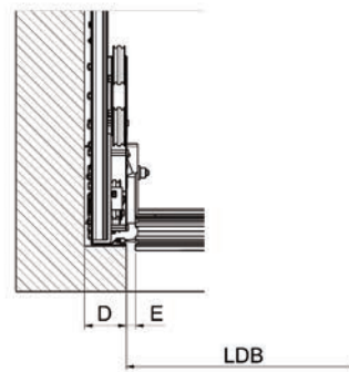
Einbau hinter der Laibung
