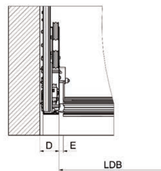
Einbau zwischen der Laibung
